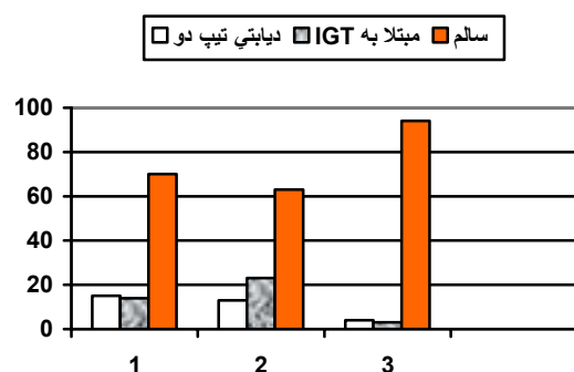
خویشاوندان مرد گروه دیابتی تیپ دو = 1، خویشاوندان مرد گروه IGT = 2، خویشاوندان مرد گروه سالم = 3 نمودار ۲. توزیع فراوانی مردان خویشاوند درجه یک افراد مورد بررسی بر حسب ابتلا به دیابت و نابرداری گلوکز
