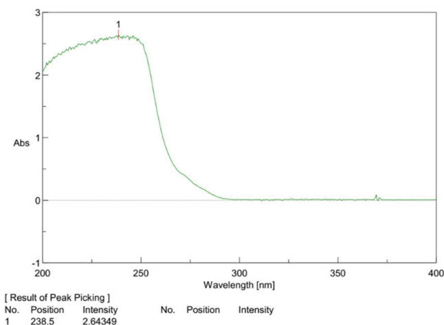
شکل ۱. اسپکتروم UV نورتریپتیلین در آب
