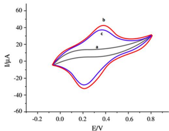
شکل ۴. ولتاموگرام چرخه‌ای به ترتیب برای: (a) الکتروود کربن شیشه‌ای اصلاح نشده، (b) الکتروود کربن شیشه‌ای اصلاح شده با نانو کامپوزیت MWCNT/C 3 O 4 و (c) الکتروود کربن شیشه‌ای اصلاح شده با GCE/MWCNT-C 3 O 4 /Hb در بافر فسفات ۰/۱ مولار
