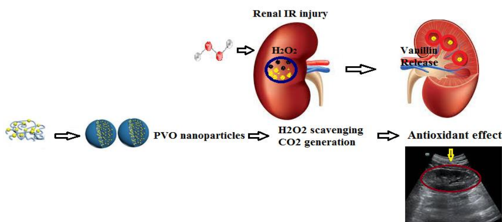
شکل ۲. نانوپارتیکل پلی وانیلین اگزالات (PVO) جهت حذف رادیکال‌های پراکسید هیدروژن ( H_2O_2 )، تصویربرداری از نواحی آسیب و تشکیل گاز دی‌اکسید کربن ( CO_2 )
