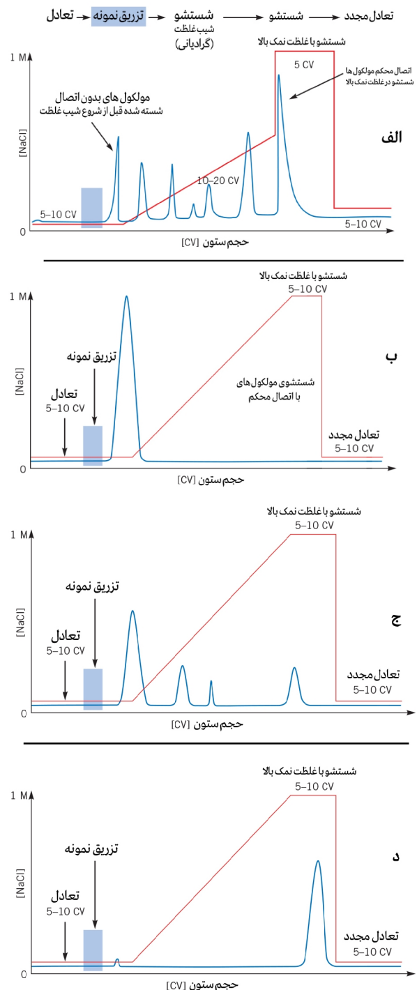
شکل ۱۰. انواع نمودارهای حاصل از کروماتوگرافی تعویض یونی [۱۶]
