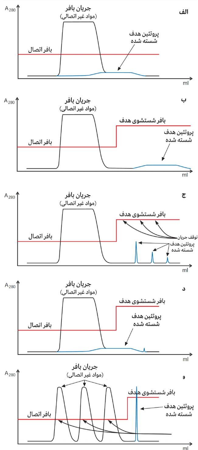
شکل ۱۳. کروماتوگرام‌های تمایلی که از وضعیت ایده‌آل در طول خالص‌سازی منحرف شده‌اند [۱۶]
