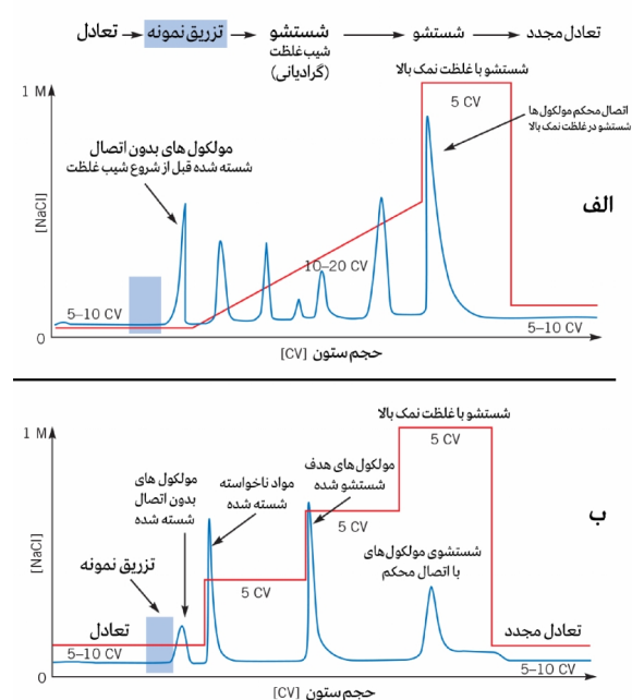
شکل ۹. کروماتوگرافی تعویض یونی [۱۶]
