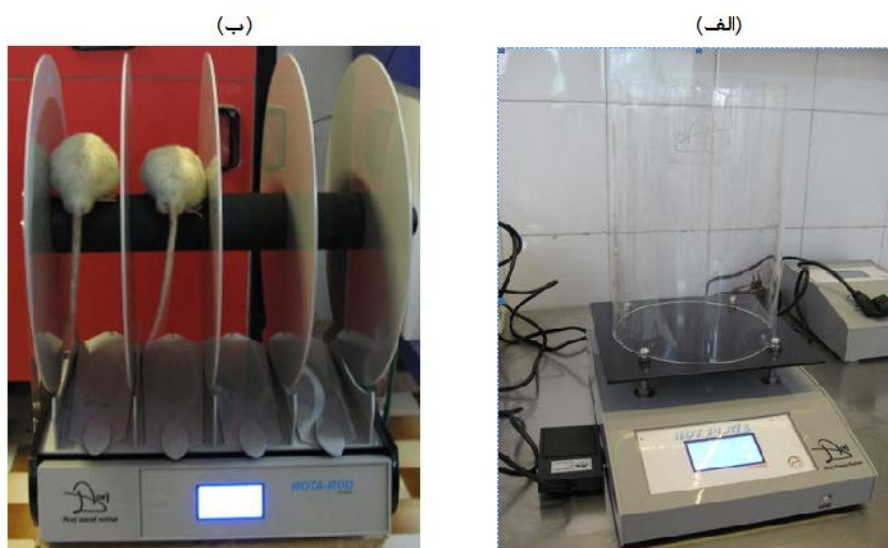
شکل ۴. الف - دستگاه آزمون صفحه داغ جهت ارزیابی اختلالات حسی و پاسخ به درد حیوانات قبل و ۲۴ ساعت پس از وقوع ایسکمی. ب - دستگاه روتارود جهت ارزیابی حس تعادل و وضعیت حرکت حیوانات قبل و ۲۴ ساعت پس از وقوع ایسکمی مغزی.
