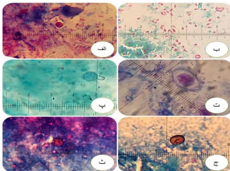
شکل ۱. رنگ آمیزی اسیدفست، ذیل نلسون و تری کروم که اووسیت‌های تک‌یاخته‌ای روده‌ای را نشان می‌دهد. الف- گونه کریپتوسپوریدیوم (ع-۶ میکرو متر) ب- میکروسپوریدیا (ع-۱ میکرو متر) پ- بلاستوسیستیس (۵۰-۱۵۰ میکرو متر) ت- ایزوسپورا (۲۵-۲۰ میکرو متر) ث- سیکلوسپورا (۱۰-۸ میکرو متر) ج- ژیا ردیا (۸-۱۴ میکرو متر)
