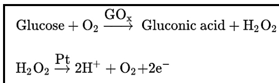
شکل ۲. نخستین سنسور الکتروشیمیایی گلوکز بر پایه Pt اصلاح شده با Gox [۹]
