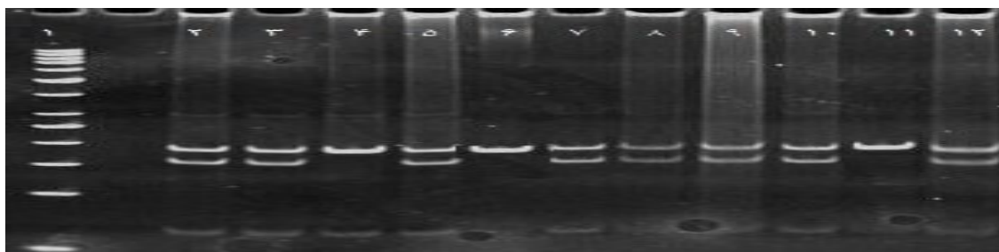
شکل ۳. الگوهای برش با آنزیم Tai 1 روی ژل پلی آکریل آمید ٪۸. ستون ۱ مارکر مولکولی plus ۵۰ bp ، ستون ۲، ۳، ۴، ۵، ۷، ۸، ۹ الگوی حساس دارای دو باند ۱۸۷ bp و ۱۵۴ bp ، ستون ۱۰، ۱۱، ۱۲ الگوی مقاوم به دارو دارای دو باند بهم چسبیده ۱۸۷ و ۱۸۵ bp ، ستون ۱۲ سوپه H37RV است.
